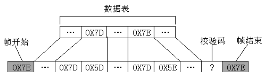
图1 数据帧封装格式
